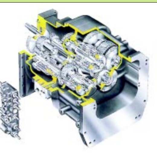
Caixa de transmissão e escalonamento de marchas do New Holland 8670
